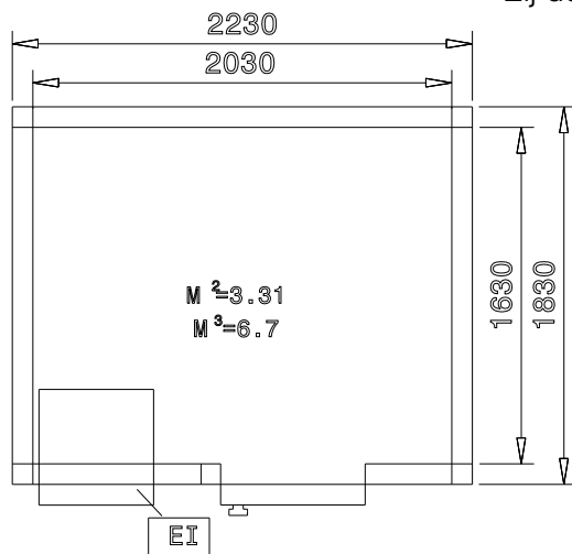
Zij aanzicht
